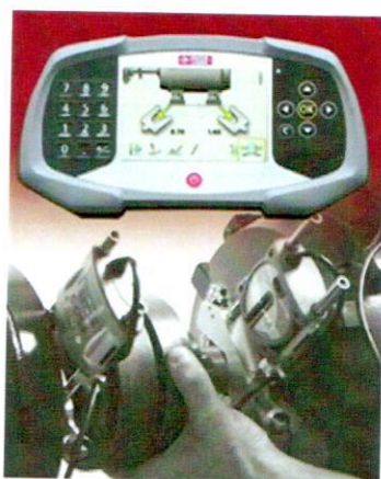
Рисунок 3 – Системы лазерные для измерения перемещений модели Fixturlaser GO Pro, Fixturlaser GO Basic
